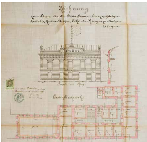
Plan Hotelu "Herz", 1879 r.; zbiory Muzeum Zamek w Oświęcimiu.
